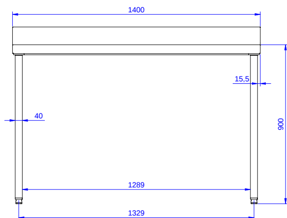
Côté
